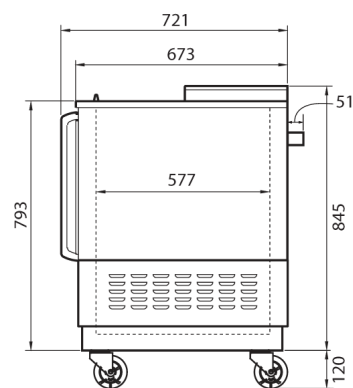
ВИД СБОКУ
